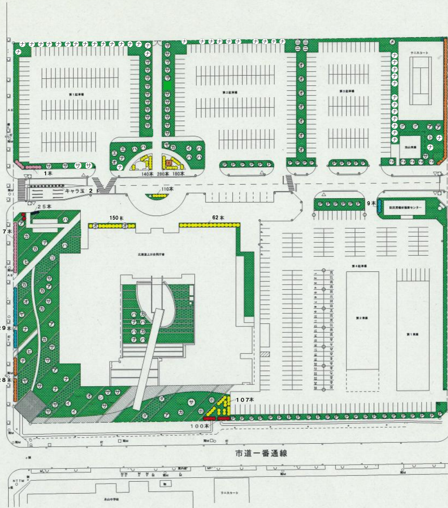
上川合同庁舎植栽平面図
