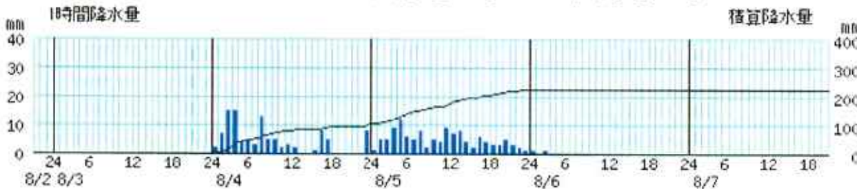
東川 (12451) 1981年8月2日21時～1981年8月7日21時
