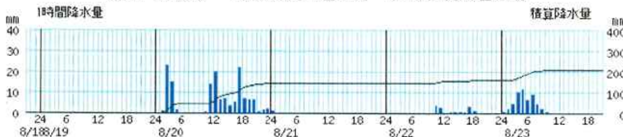
東川 (12451) 2005年8月19日21時～2005年8月24日21時
