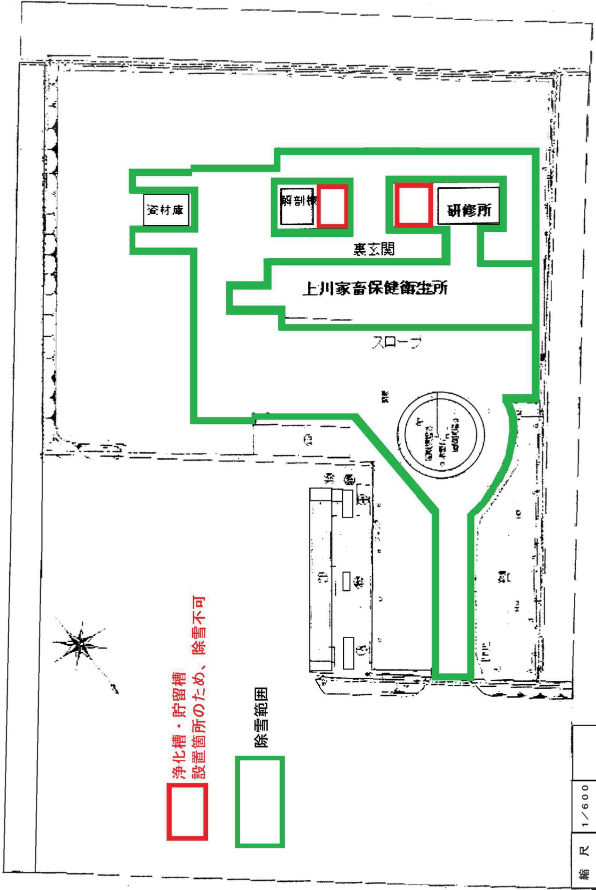
上川家畜保健衛生所平面図(除雪用)
